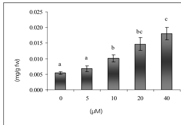
شکل ۱- تغییر محتوای آنتوسیانین‌های برگ در گیاه نعناع تحت تیمار غلظتهای مختلف فلز روی ( p < 0.05 )
