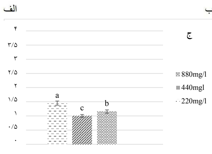
شکل ۶- الف) منحنی ذوب، ب) تکثیر و ج) نمودار تفاوت در میزان بیان ژن 4CL در تیمارهای مختلف گیاه بادرنجبویه
