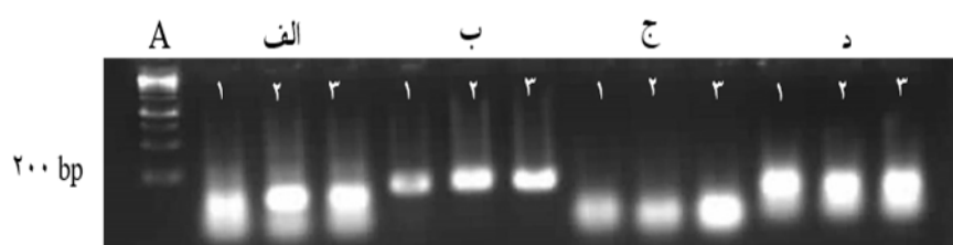
شکل ۴- درستی سنتز cDNA و آغازگرهای طراحی شده؛ (A) خط کش، (الف) توبولین، (ب) 18S rRNA، (ج) PAL و (د) 4CL در تیمارهای مختلف گیاه بادرنجبویه شامل: (۱) ۲۲۰ mg/L؛ (۲) ۴۴۰ mg/L و (۳) ۸۸۰ mg/L کلسیم کلراید
