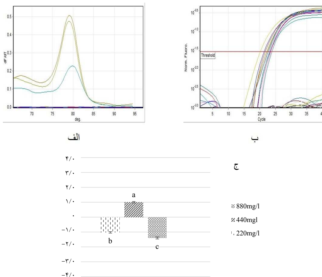
شکل ۵- الف) منحنی ذوب، ب) تکثیر و ج) نمودار تفاوت در میزان بیان ژن PAL در تیمارهای مختلف گیاه بادرنجبویه با استفاده از تکنیک qRT-PCR
