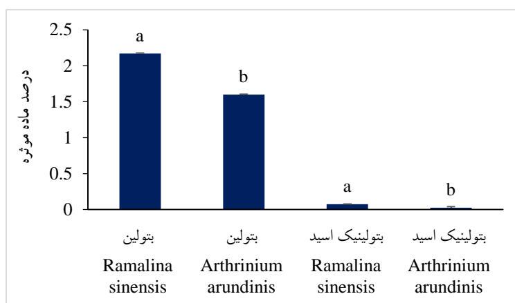
شکل ۵- نمودار مقایسه میانگین میزان ماده مؤثره در بافت گل‌سنگ R. sinensis و قارچ جدا شده از آن ( A. arundinis )
