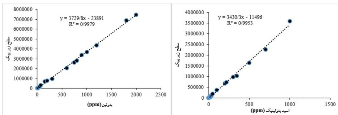
شکل ۴- منحنی کالیبراسیون اسید بتولینیک و بتولین
