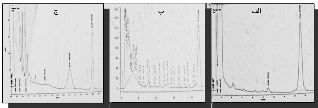
شکل ۳- منحنی کروماتوگرام، الف: استاندارد (اسید بتولینیک و بتولین)؛ ب: گل‌سنگ ( R. sinensis ) و قارچ جدا شده از آن ( A. arundinis )
