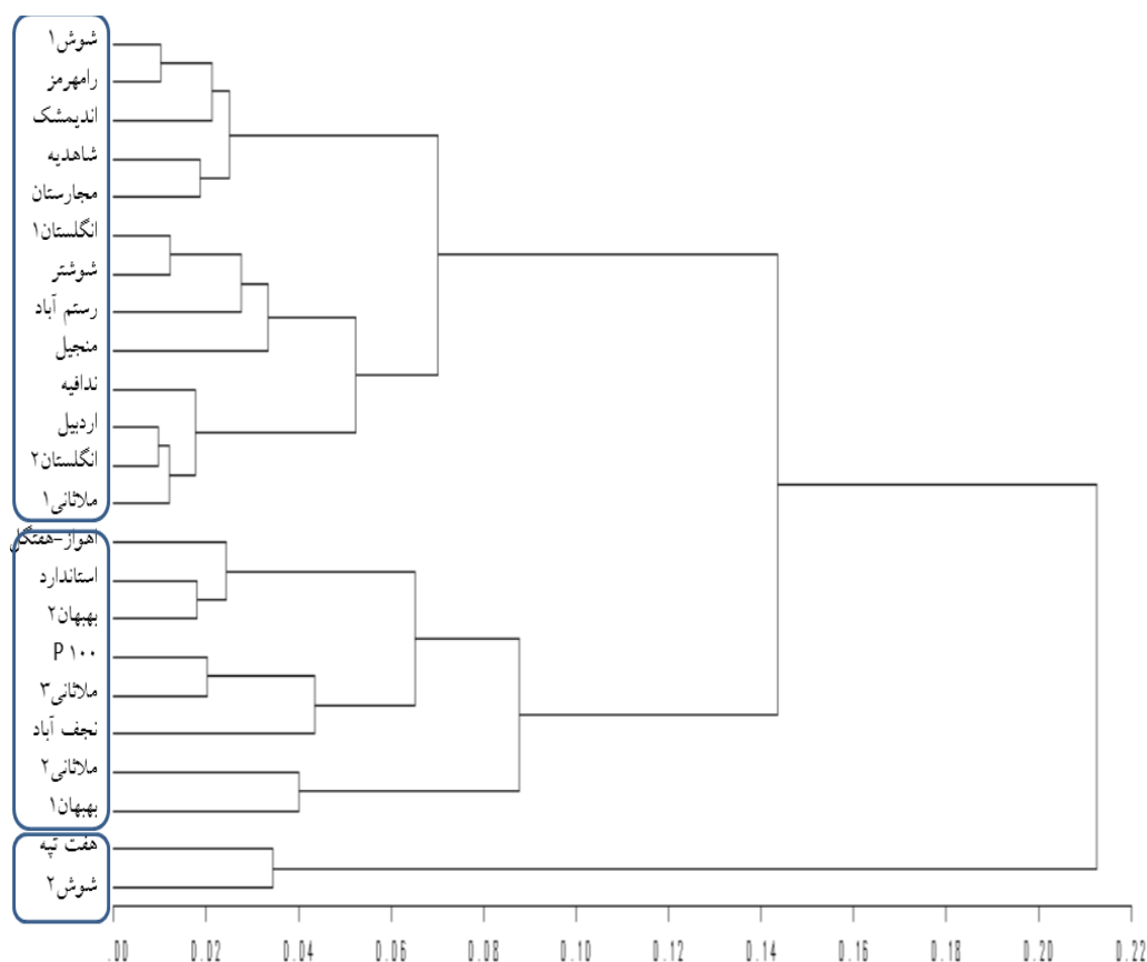
شکل ۱- دندروگرام حاصل از تجزیه خوشه‌ای براساس فاصله مربع اقلیدسی و الگوریتم وارد
