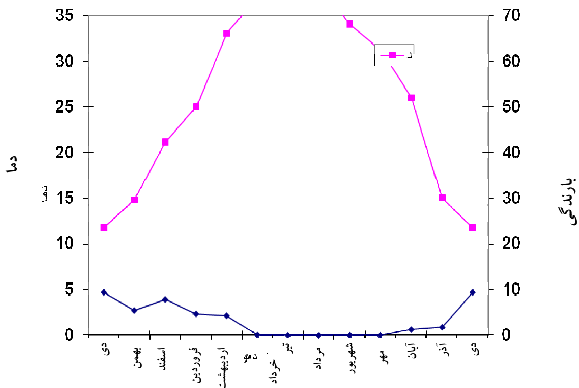
شکل ۱- منحنی آمبروترمیک ایستگاه هواشناسی شهداد
